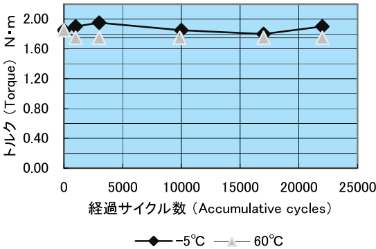
OWH8－2.0NRW 信頼性試験データ (高低温環境) OWH8-2.0NRW Reliability test data
