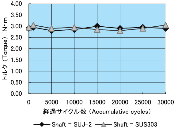
OWH10－3.0NRW 信頼性試験データ (常温) OWH10-3.0NRW Reliability test data
