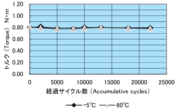
OWH8－0.8NRS 信頼性試験データ (高低温環境) OWH8-0.8NRS Reliability test data
