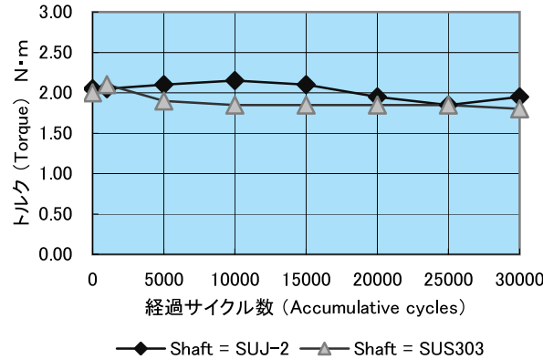
OWH8－0.8NRS 信頼性試験データ (高低温環境) OWH8-0.8NRS Reliability test data
